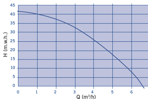
Krzywa wydajności
