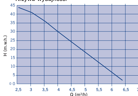
Krzywa wydajności
