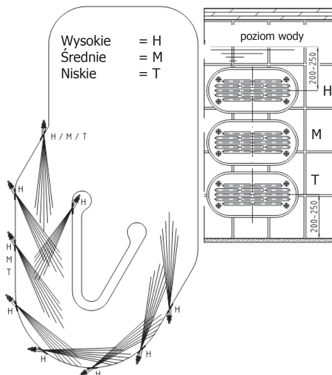
Typowa instalacja
