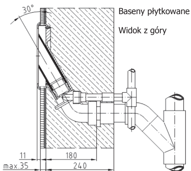
Typowa instalacja
